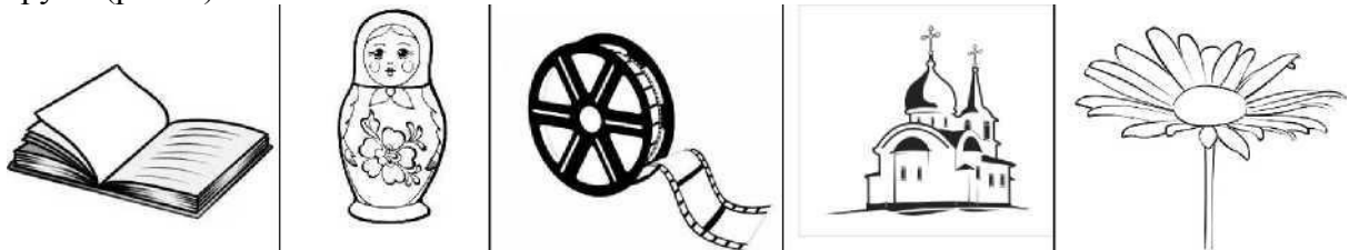
Рис. 1. Примеры картинок
